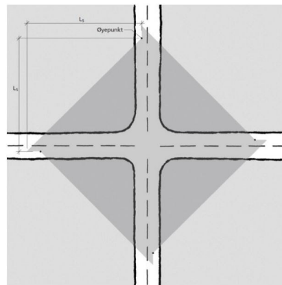
Figur E.9: Sikt i uregulerte X-kryss
