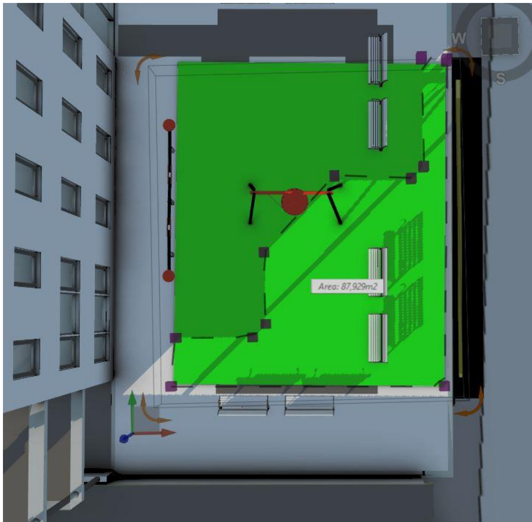
21. mars kl.15. Soldekning leikeplass.
